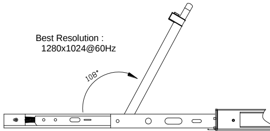
图 3-4 控制平台翻开角度
