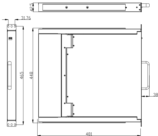
图 1-1 整体外观尺寸图
