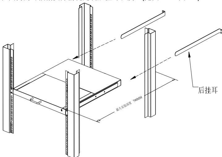
图 2-1 机架安装图(一)
