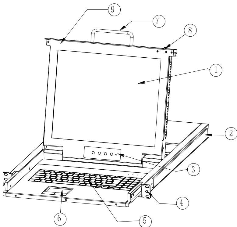
前视图 (见图 1-2)
