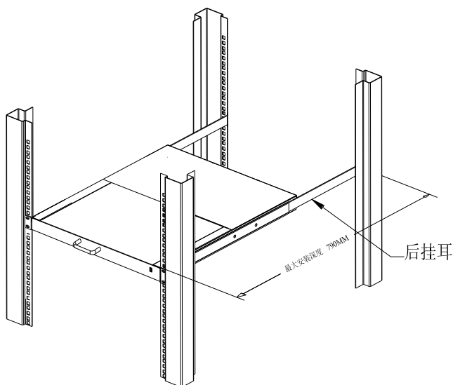
图 2-2 机架安装图(二)
