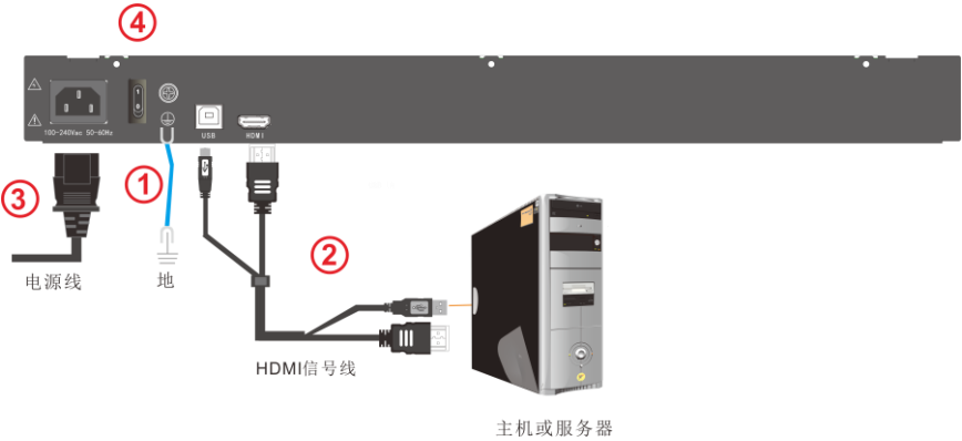
图 3-2 连线方式
